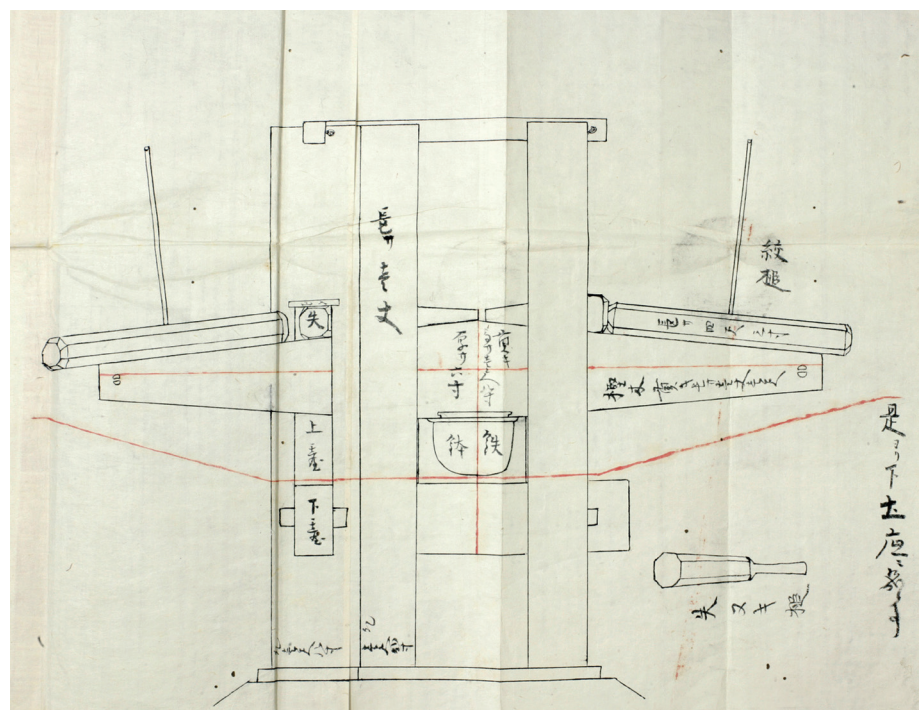
* 毛利家文庫 58絵図649「製蠟板場道具絵図」
